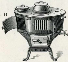
Buanderie cuisinière
