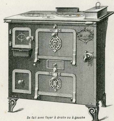
Se fait avec foyer à droite ou à gauche
